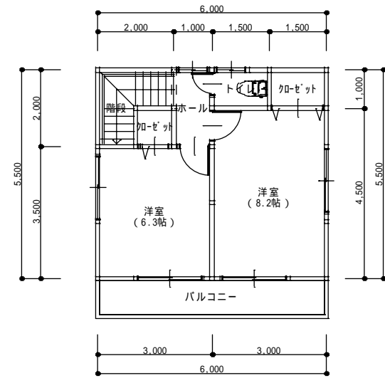
3階 平面図 S:1/100
